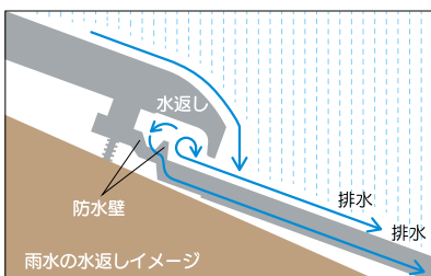
雨水の水返しイメージ
